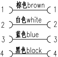
接线图 Circuit diagram
