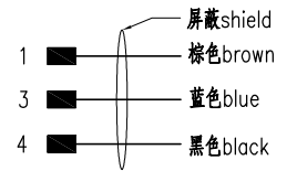
接线图 Circuit diagram
