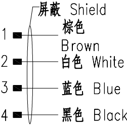
接线图 Circuit diagram
