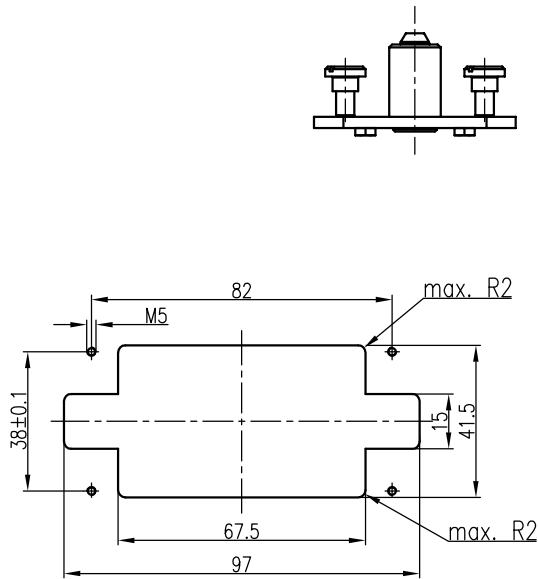
安装开孔图 Panel cut out
