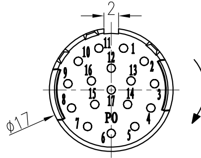
触点排列: 配合面 Contact arrangement: mating side
