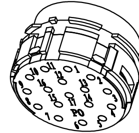
触点排列: 配合面 Contact arrangement: mating side
