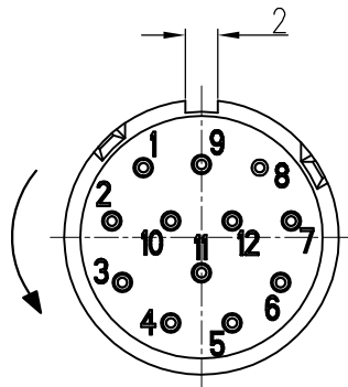
触点排列: 配合面 Contact arrangement: mating side
