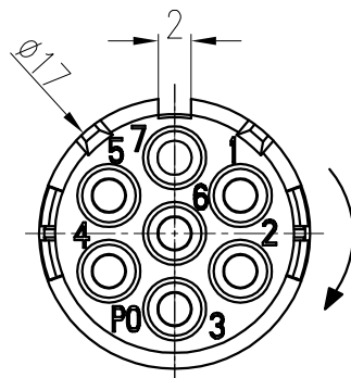
触点排列: 配合面
