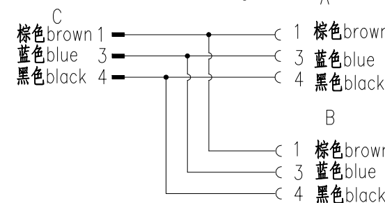
接线图 Circuit diagram
