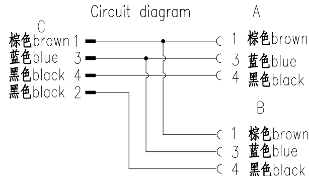
接线图
