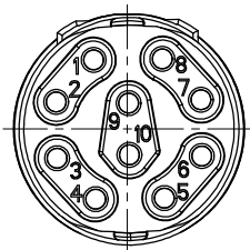
孔位图 比例2: 1
