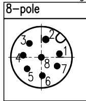
针位排布图
