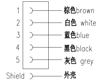
接线图 Circuit diagram
