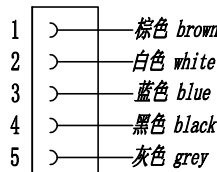
接线图 Circuit diagram
