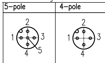
针位排布图
