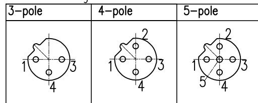
针位排布图
