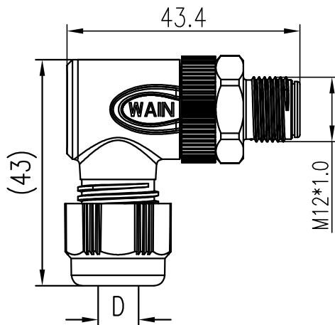
电缆直径:D6,D8 Cable outlet:D6,D8
