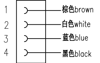
接线图 Circuit diagram
