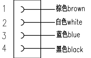
接线图 Circuit diagram
