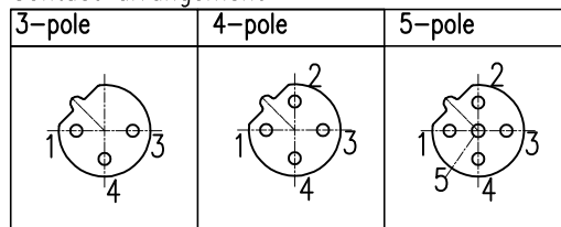
针位排布图
