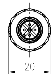
电缆直径:2D5 Cable outlet:2D5
