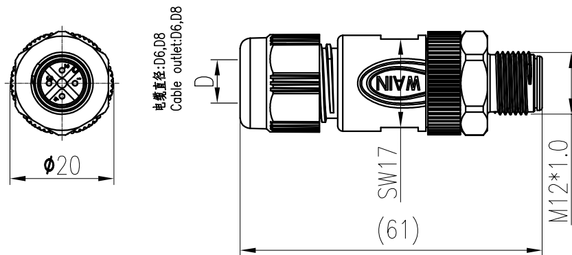
针位排布图
