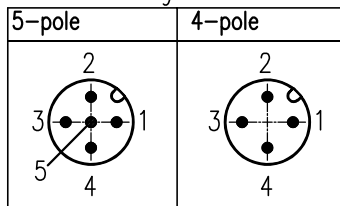
针位排布图
