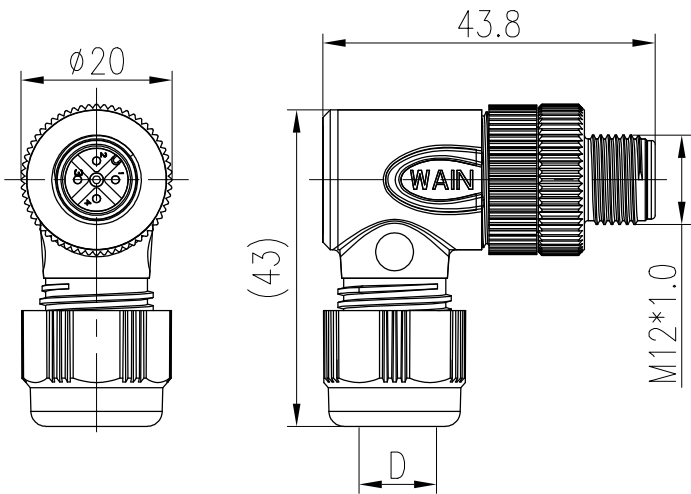
电缆直径: D6, D8 Cable outlet: D6, D8
