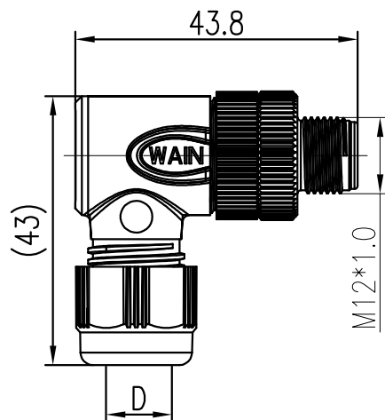
电缆直径: D6, D8 Cable outlet: D6, D8
