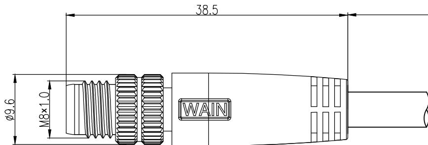
针位图 Contact arrangements 4Pin
