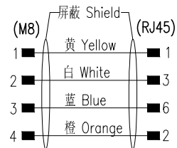
接线图 Circuit diagram
