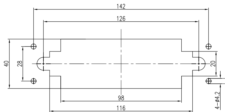
开孔尺寸图
