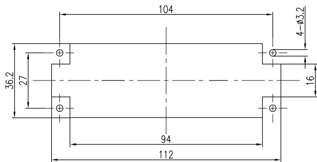
开孔尺寸图
