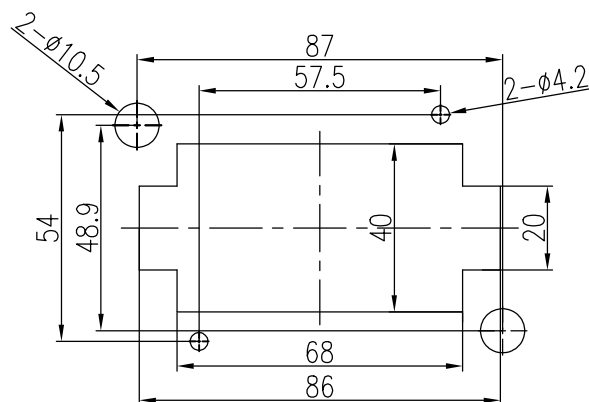
开孔尺寸图 (Paenl cut out)
