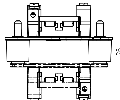
插合距离26mm
