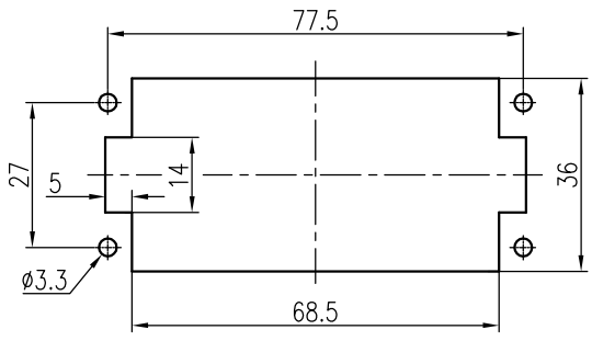
面板安装孔图 Panel cut out
