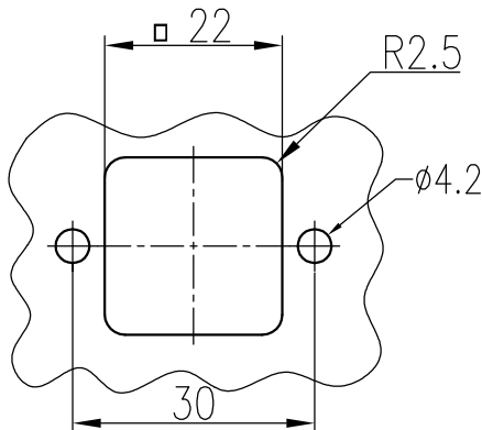
面板开孔图
