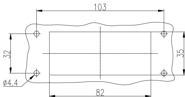
面板开孔图
