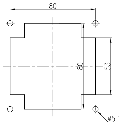
面板开孔图
