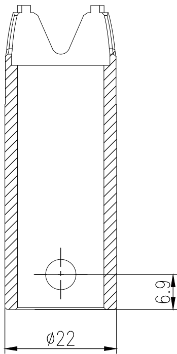
截面 A-A
