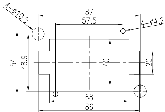
开孔尺寸图 (Paenl cut out)
