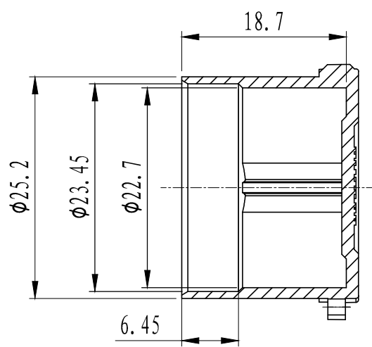
截面 A—A
